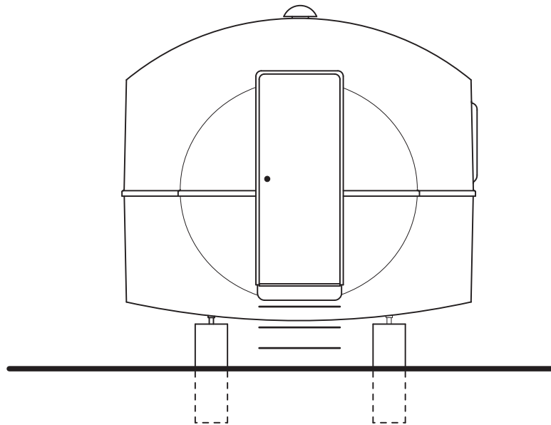
Ansicht Eingang M 1 : 50
